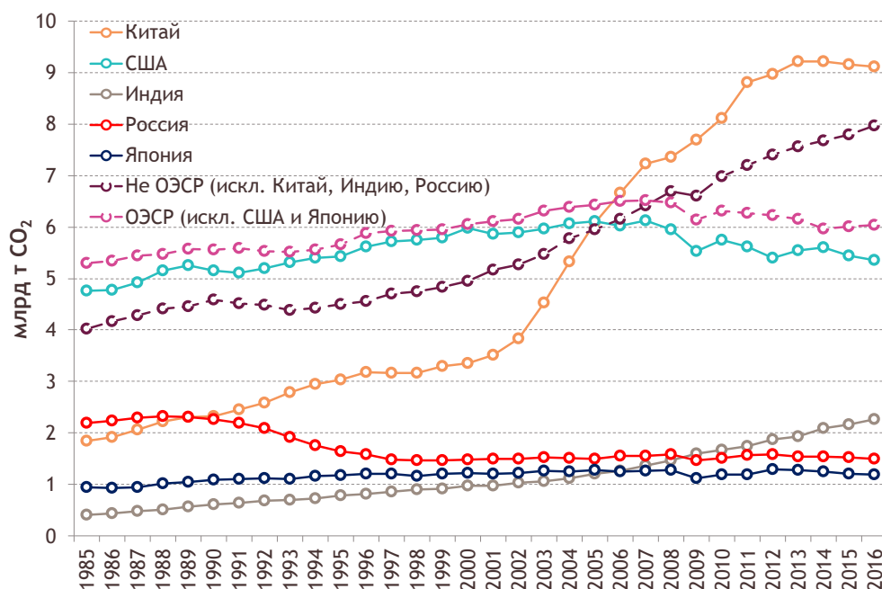
Выбросы CO 2 по ведущим странам и регионам мира, 1985-2016 годы
